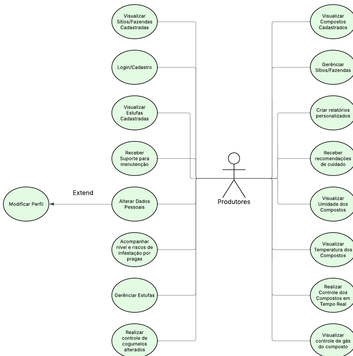
Figura 7: Diagrama de Casos de Uso – Selene
