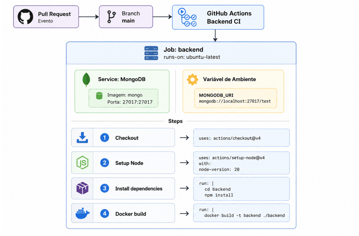
Figura 16: Modelo CI - Selene
