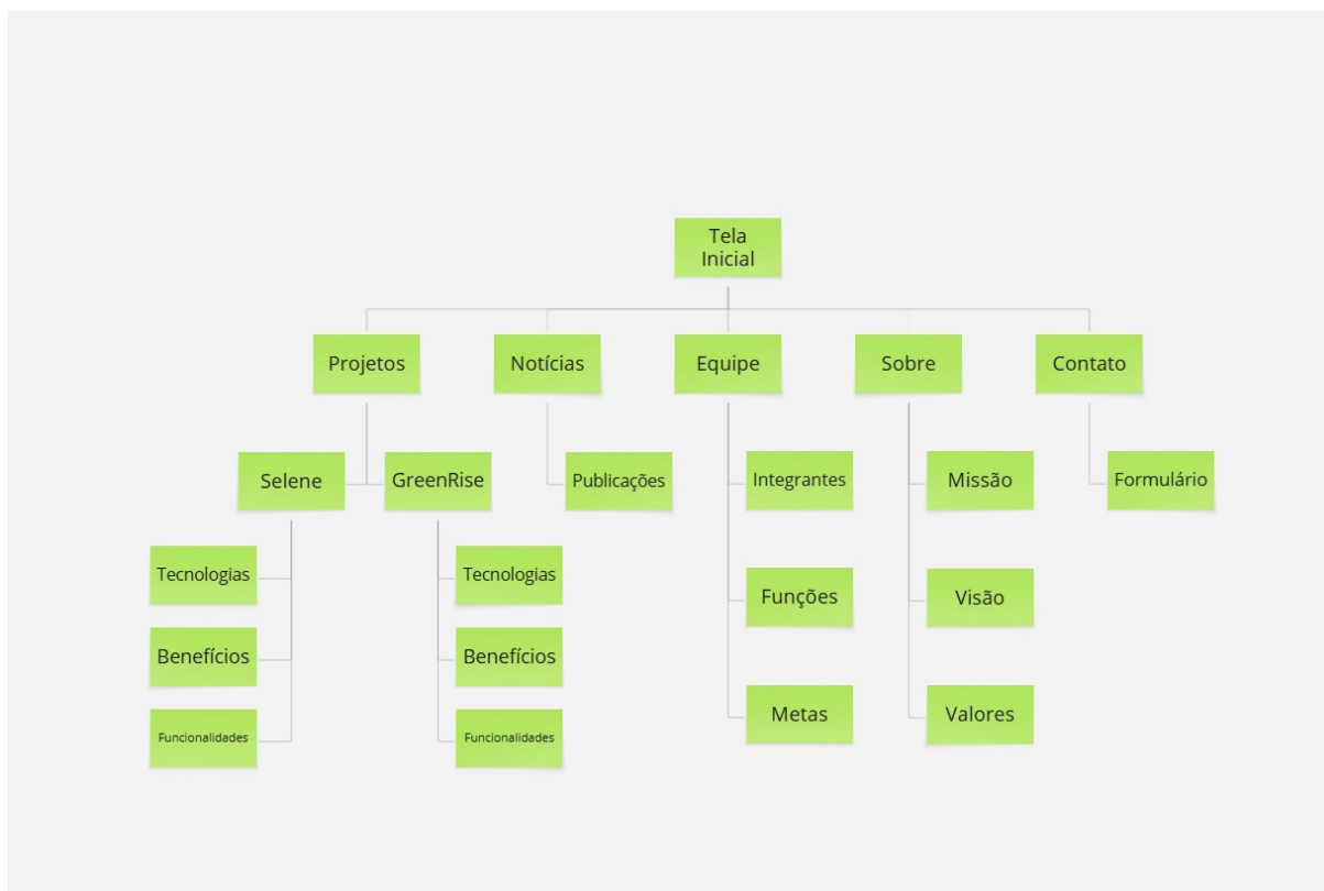
Figura 5: Sitemap do Projeto Selene
