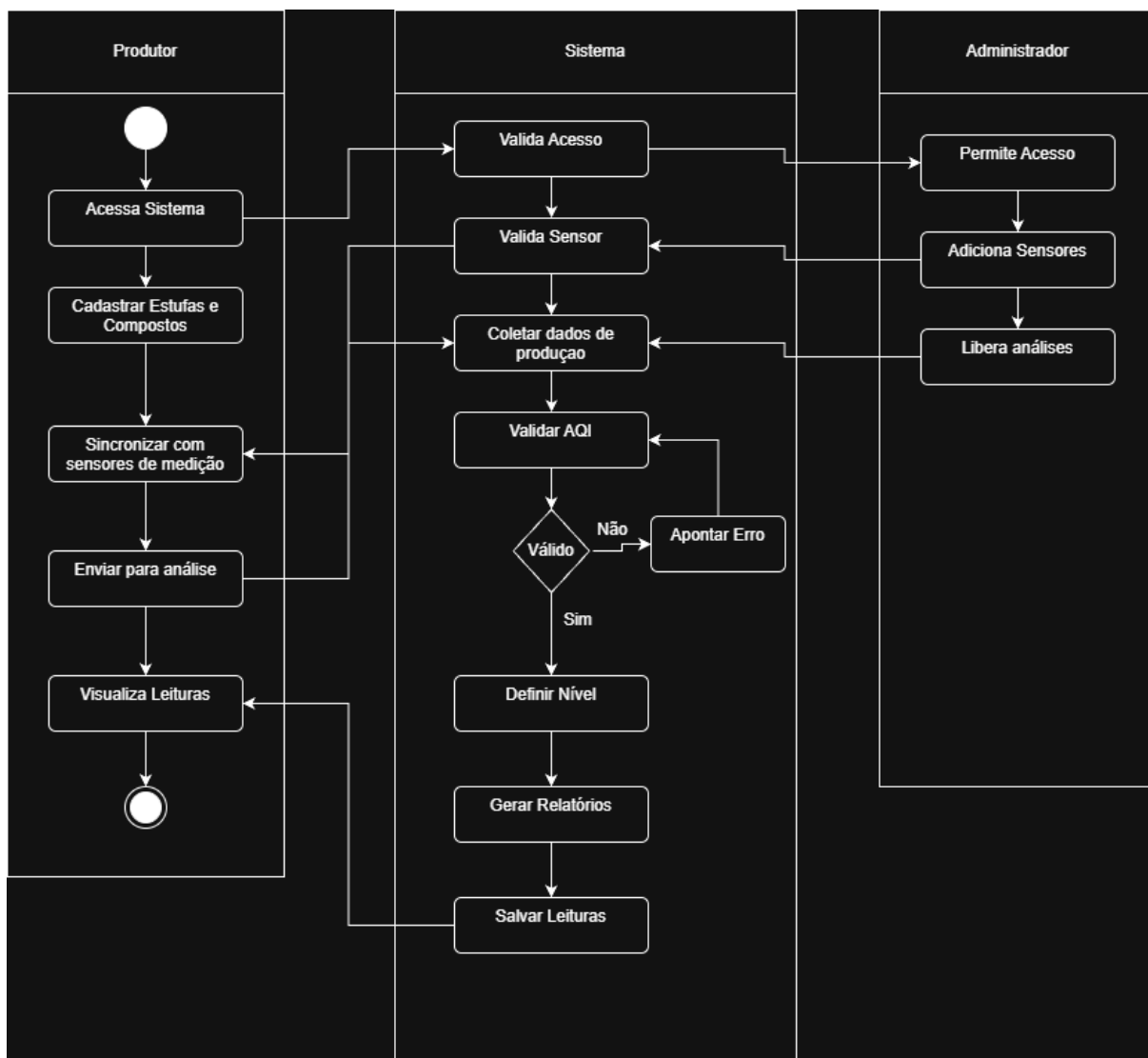
Figura 11: Diagrama de Atividades – Selene
