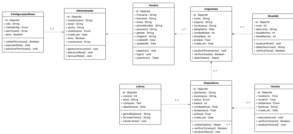
Figura 8: Diagrama de Classes – Selene
